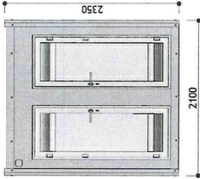
ÖN CEPHE
